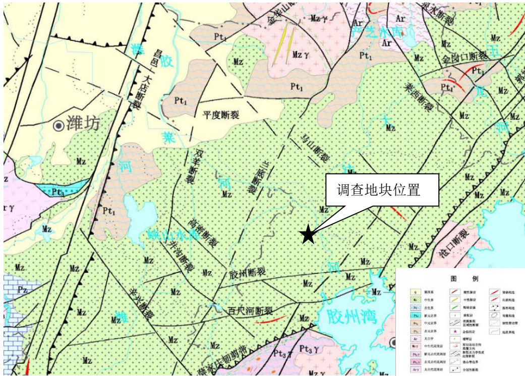
图 3.1-2 区域构造地质图 (1:50 万)
